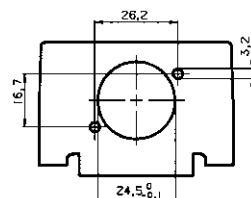
Audio-Steckbuchse XLR
