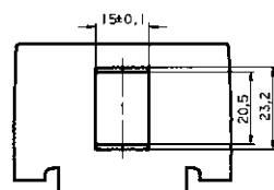
Modular Jack Kat. 5
