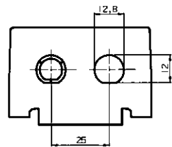
BNC/TNC 2xBNC/TNC-Kabeleinbaubuchse oder 2xTNC-Einbaubuchse, 1 Öffnung ausbrechbar
