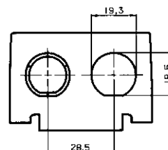
Twinax
