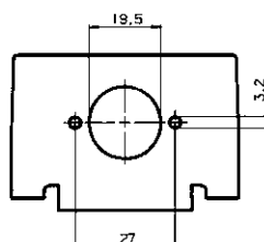
Audio-Stecker XLR
