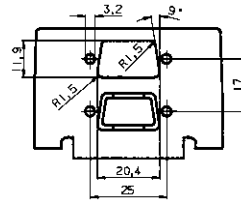
D-Sub 9polig
