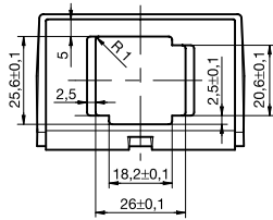
IBM-LAN 4-poliger Datenstecker für IBM-LAN z.B. AMP-Typ 554000-1
