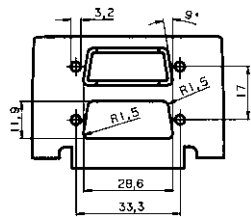
D-Sub 15polig
