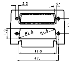
D-Sub 25polig
